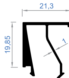
4312 | Ağırlık - Weight 0,237 Kg/Mt
