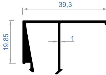
4309 | Ağırlık - Weight 0,303 Kg/Mt
