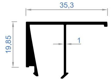
4310 | Ağırlık - Weight 0,283 Kg/Mt
