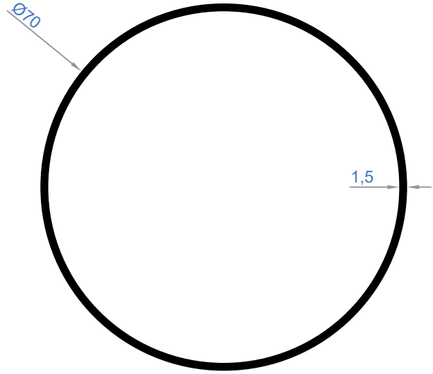
4307 | Ağırlık - Weight 0,875 Kg/Mt
