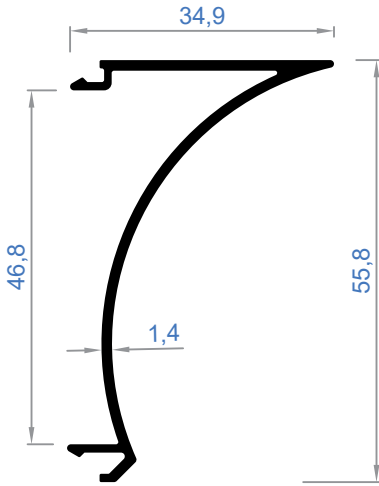
4306 | Ağırlık - Weight 0,418 Kg/Mt
