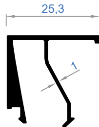
4311 | Ağırlık - Weight 0,251 Kg/Mt
