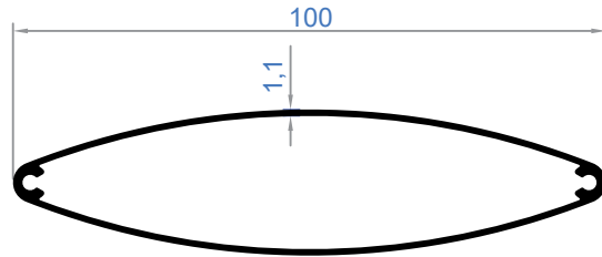
3506 | Ağırlık - Weight 0,678 Kg/Mt
