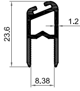
1409 | Ağırlık - Weight 0,224 Kg/Mt
