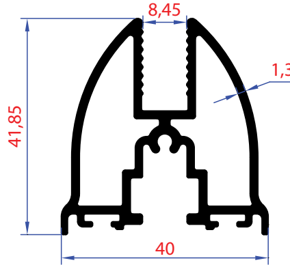
1411 | Ağırlık - Weight 0,822 Kg/Mt
