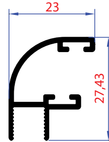
1413 | Ağırlık - Weight 0,270 Kg/Mt
