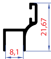
1407 | Ağırlık - Weight 0,137 Kg/Mt
