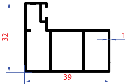
1414 | Ağırlık - Weight 0,488 Kg/Mt
