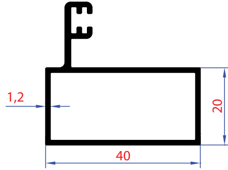
1405 | Ağırlık - Weight 0,464 Kg/Mt
