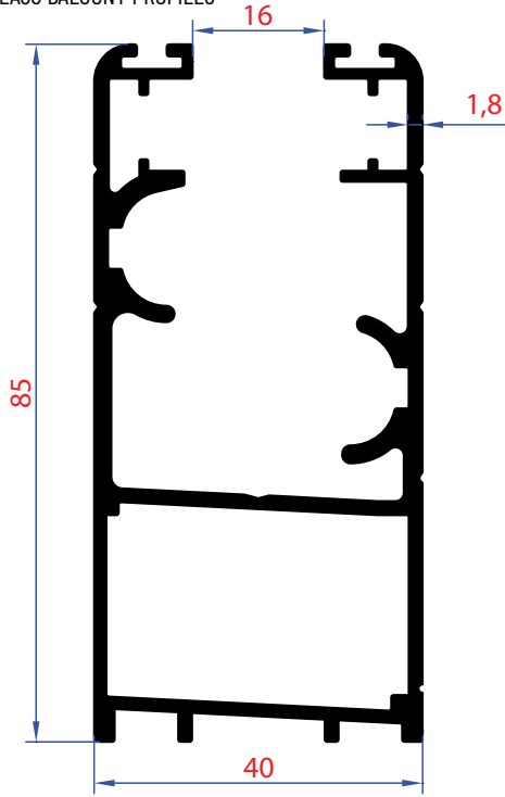
1401 | Ağırlık - Weight 1,641 Kg/Mt
