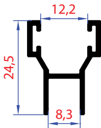
1406 | Ağırlık - Weight 0,221 Kg/Mt
