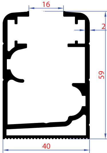
1404 | Ağırlık - Weight 1,250 Kg/Mt
