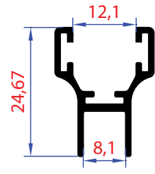
1408 | Ağırlık - Weight 0,224 Kg/Mt
