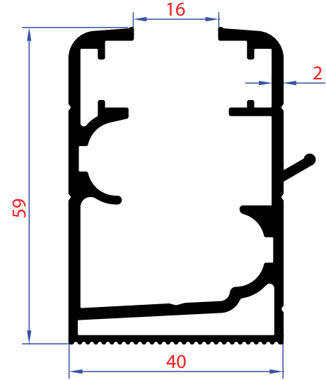
1403 | Ağırlık - Weight 1,277 Kg/Mt
