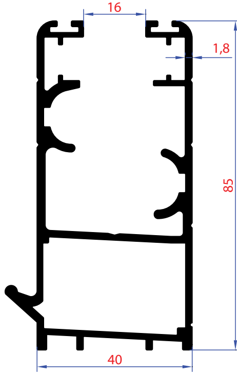
1402 | Ağırlık - Weight 1,693 Kg/Mt
